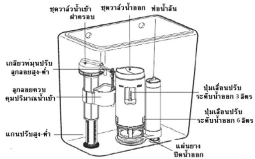
ภาพประกอบรายละเอียดของฟลั้ววาล์วชนิด 2 ปั๊ม
