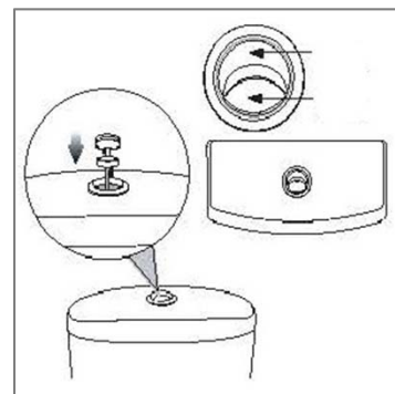
7. ตรวจสอบทิศของปุ่มกด
