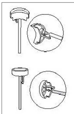
6. ประกอบก้านเข้ากับปุ่มกด
